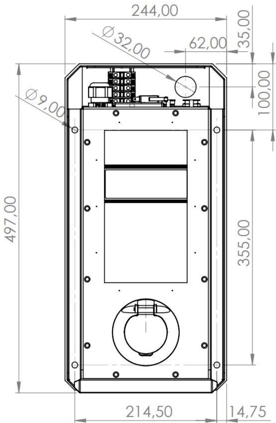
Рис. 3.1 Установочні розміри 3C EFC AC-32J2M1SB
